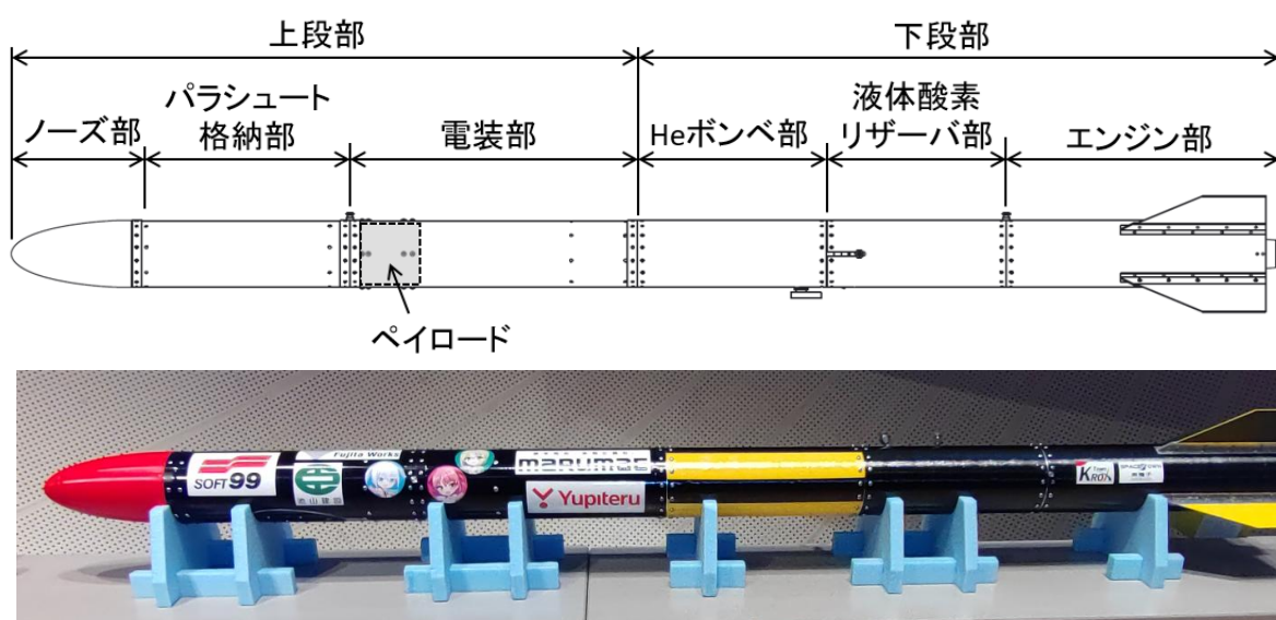
図1 6号機の外観（令和8年2月12日 機体・ペイロード公開時）
